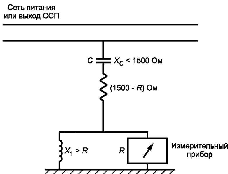
Рисунок А.1 — Схема измерений напряжения помех на зажимах сети питания или выходе ССП
