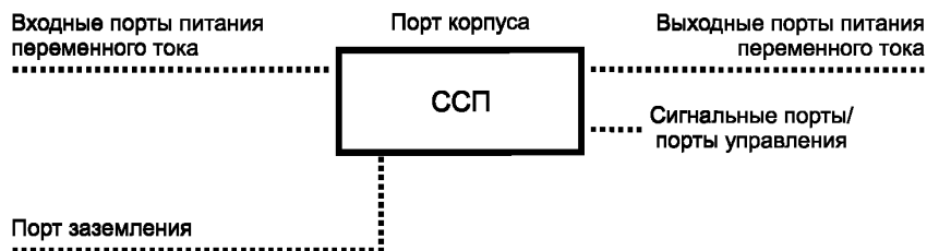
Рисунок 1 — Примеры портов
