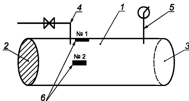
Рисунок А.1 — Трубчатый образец для тарировки акустического метода определения напряженного состояния
