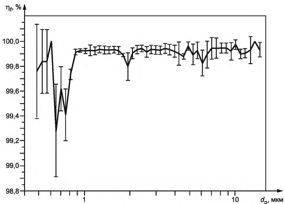
Рисунок А.2 — Характеристические кривые фильтрования для поликарбонатных фильтров (номинальной тонкостью фильтрации 0,8 мкм, диаметром 80 мм) при расходе воздуха 3 м 3 /ч — приведенные значения получены при линейной скорости потока воздуха через фильтр v = 217 мм/с
