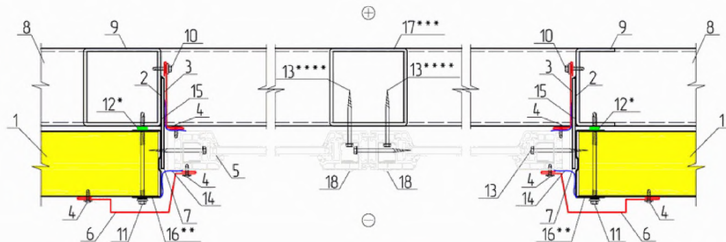
КРЕПЛЕНИЕ ОКОННОГО БЛОКА В1.4
