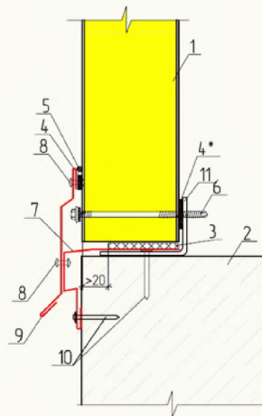
ЦОКОЛЬНЫЙ УЗЕЛ В2.4
