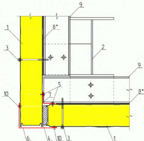
УГОЛ ЗДАНИЯ НАРУЖНЫЙ В3.2
