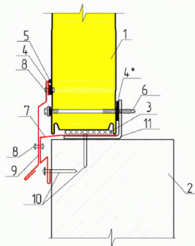
ЦОКОЛЬНЫЙ УЗЕЛ Г2.2
