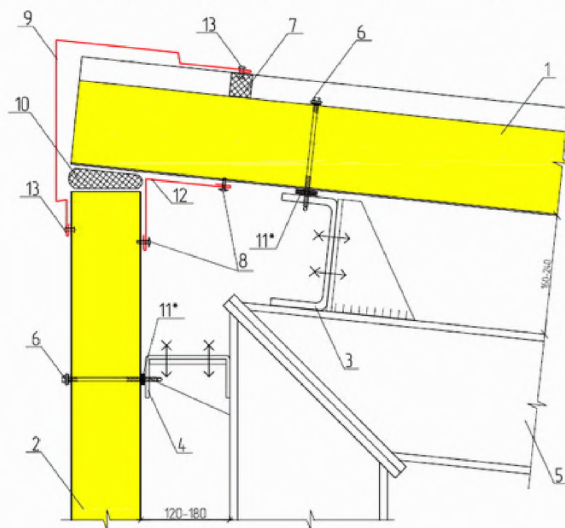
КОНЁК ОДНОСКАТНОЙ КРОВЛИ К2.1
