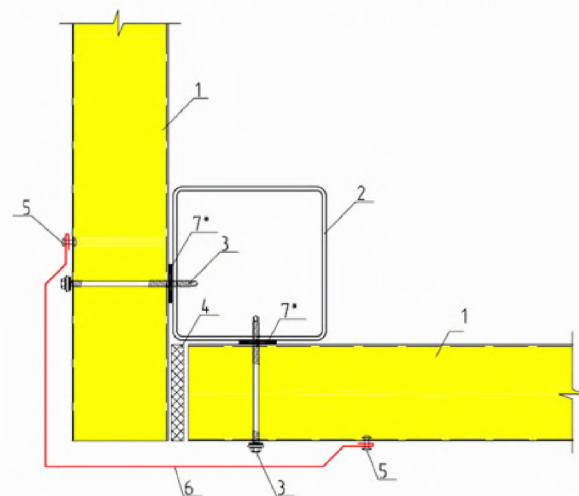
УГОЛ ЗДАНИЯ НАРУЖНЫЙ ГЗ.1
