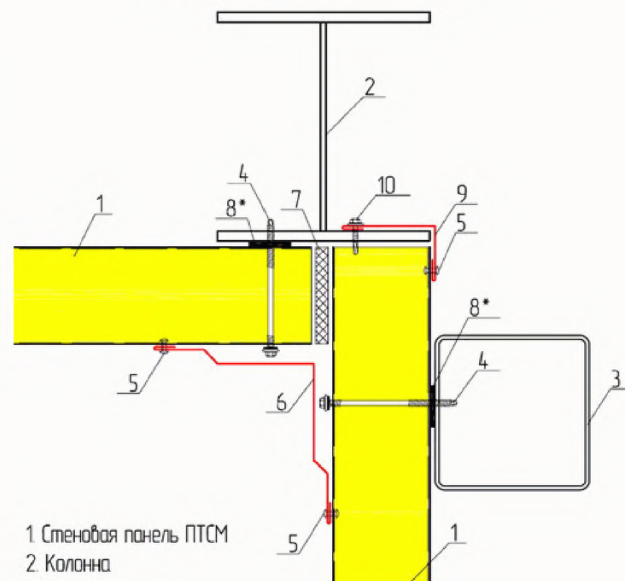
УГОЛ ЗДАНИЯ ВНУТРЕННИЙ Г4.2
