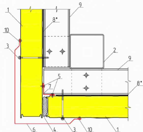
УГОЛ ЗДАНИЯ НАРУЖНЫЙ ВЗ.1
