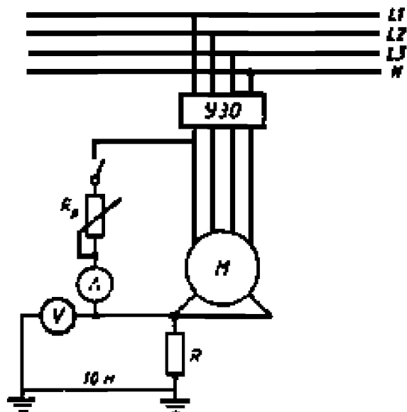
Рис.44. Схема проверки УЗО по методу 3.
