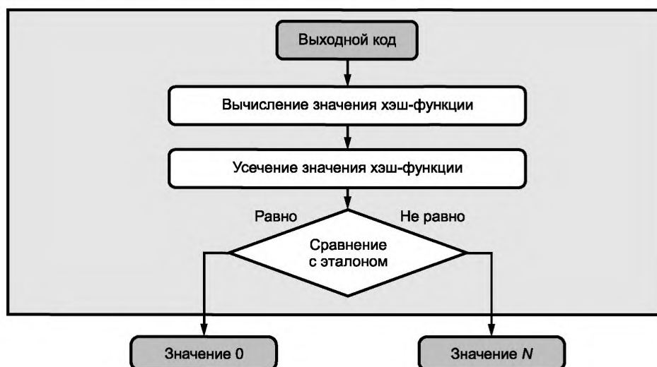
Рисунок 4 — Блок-схема работы жесткого индикатора
