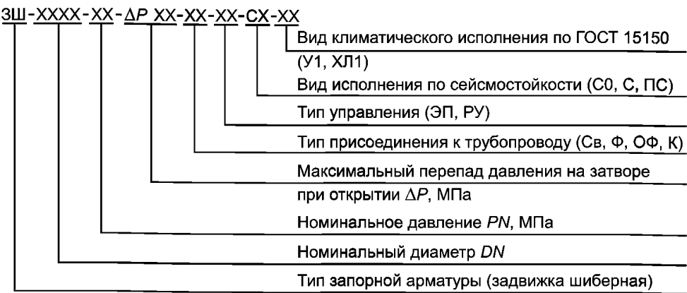
Рисунок 1 — Схема условного обозначения задвижек
