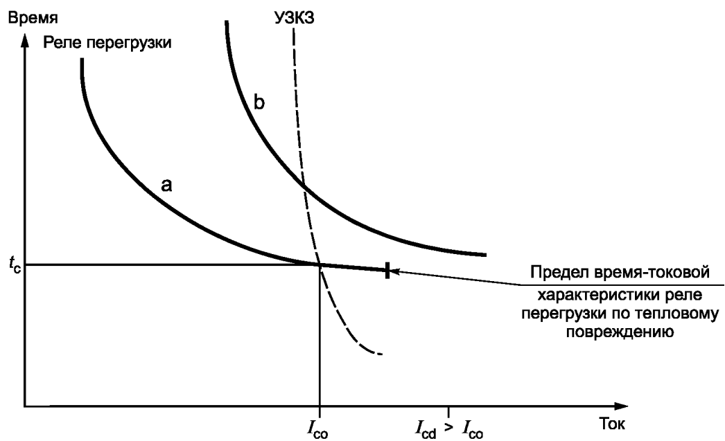
а — средняя время-токовая характеристика реле перегрузки из холодного состояния; b — время-токовая характеристика перегрузочной способности контроллера
