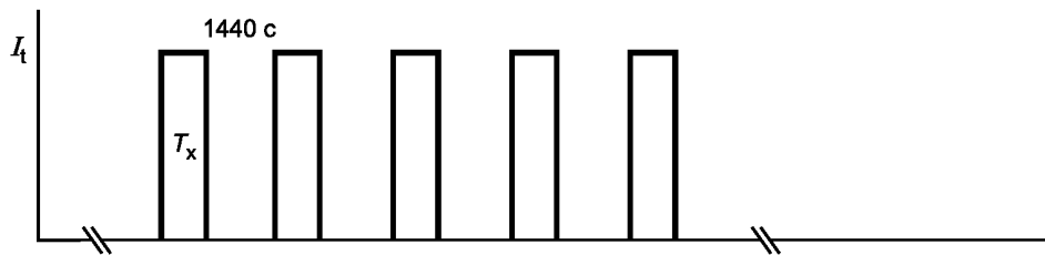
Профиль испытательного тока для AC-52b, AC-53b, AC-58b
