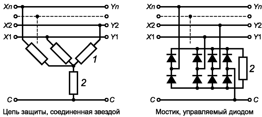
X1, X2, X_n — вводные выводы; Y1, Y2, Y_n — защищаемые вводные выводы; C — общий вывод; 1 — индивидуальный защитный элемент; 2 — общий защитный элемент
