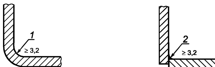
1 – радиус, образованный механической обработкой фасонным резцом; 2 – радиус, образованный сварным швом
