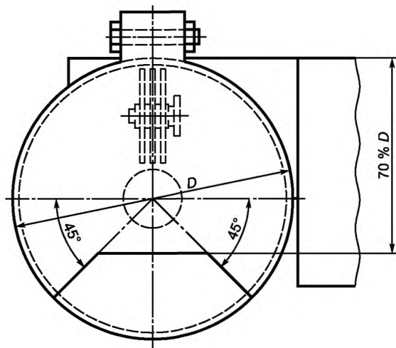
Рисунок 4 – Пример конструкции куттера типа 1
