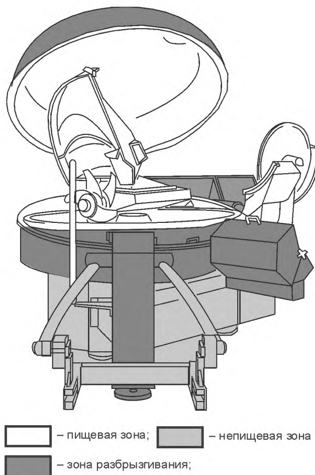
Рисунок 10 – Гигиенические зоны куттера типа 2
