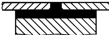
Рисунок А.9 — Пищевая зона. Непрерывный шов с плоской лицевой поверхностью и накладкой
