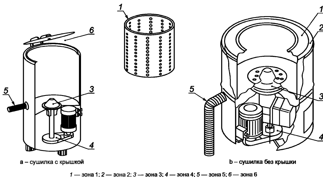
Рисунок 2 — Опасные зоны сушилки
