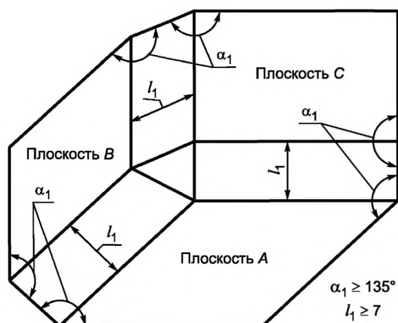
Рисунок А.4 — Соединение поверхностей в пищевой зоне
