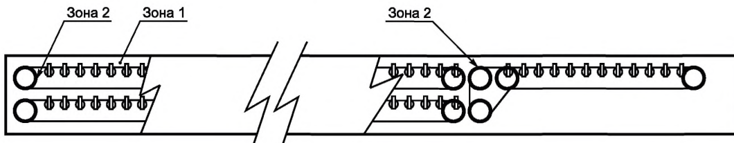
Рисунок 3 — Опасные зоны транспортера механизма возврата и накопителя бастунов
