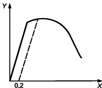
X — деформация, % Y — механическое напряжение, МПа
