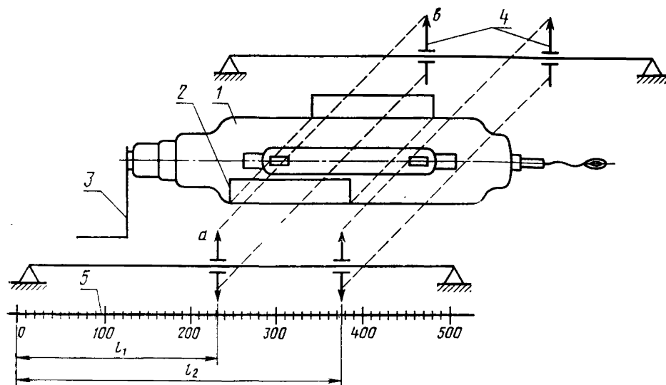
1—лампа; 2—основание; 3—упор; 4—визирное устройство; 5—шкала отсчета
