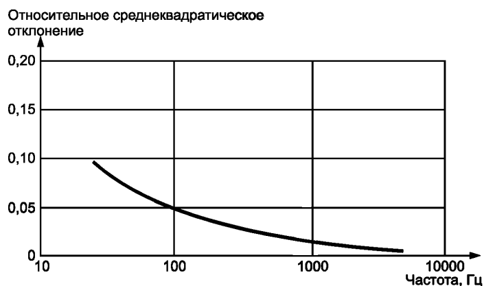
Рисунок 1 — Пример определения среднеквадратического отклонения
