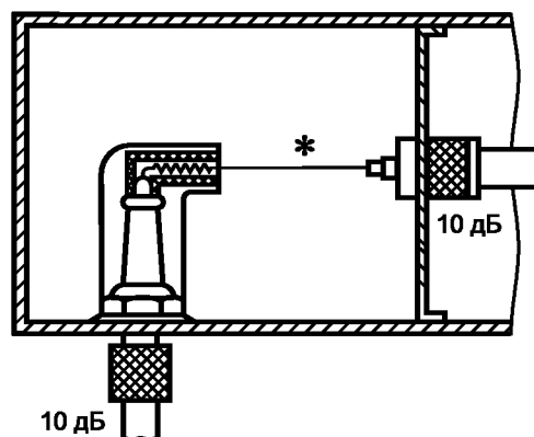
Рисунок Е.6 — Прямоугольное помехоподавляющее устройство системы зажигания со свечой зажигания (экранированное или неэкранированное)
