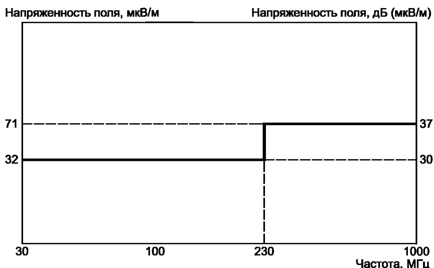
Рисунок 4 — Нормы радиопомех (детектор средних значений) для расстояния 10 м
