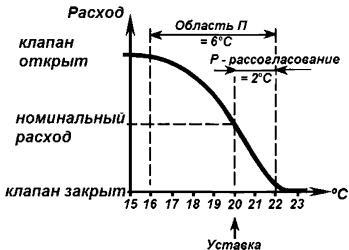
Рисунок 7.5 – Характеристика термостатического вентиля
