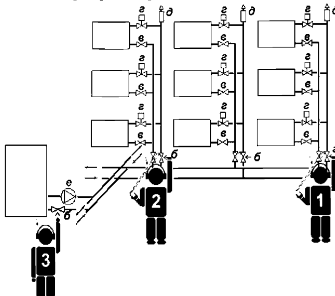
a – эталонный клапан балансировочный; б – клапаны-партнеры балансировочные; в – запорно-регулирующий клапан; з – термостатический клапан; д – воздухоотводчик; е – насос
