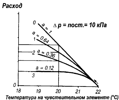
Рисунок 7.8 – Характеристики открытия термостатического вентиля с регулировкой через дополнительное гидравлическое сопротивление при различных настройках (кривые 0, 1, 2, 3)
