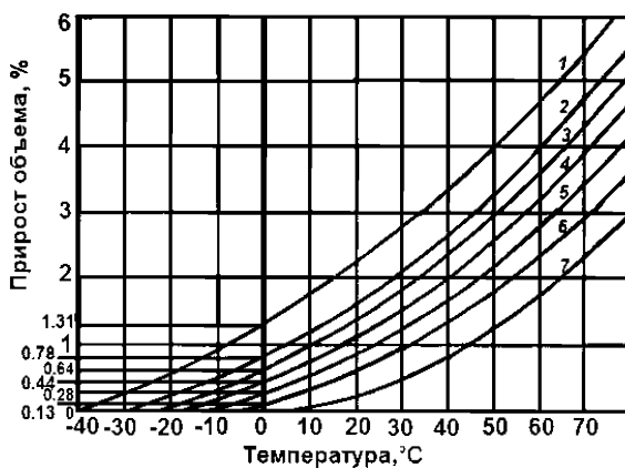
Рисунок 7.2 – Температурное расширение воды при ее нагреве (охлаждении) от 10 °С до средней температуры системы
