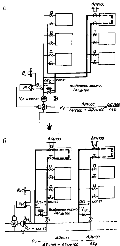
Рисунок 7.7 – Расчет авторитета клапана на примере 2-х систем
