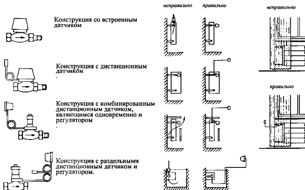
Рисунок 7.4 – Типы конструкции термостатического вентиля и варианты размещения датчика
