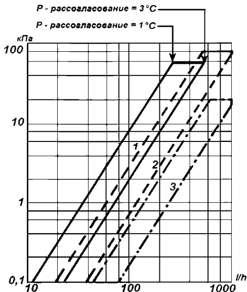
Рисунок 7.6 – Характеристики термостатических вентилей трех серий с одинаковым условным проходом
