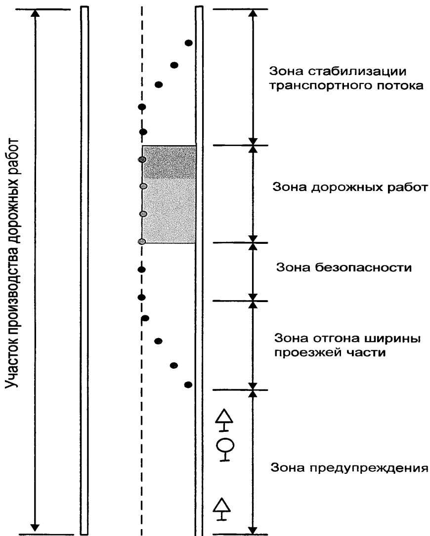
Рисунок 1 – Зонирование места дорожных работ
