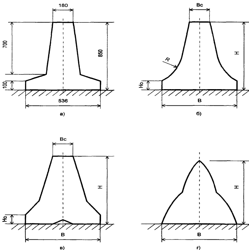
а) – типовое временное бетонное ограждение ЗР 200.86.54 ТУ 5899-066-03984346-2011; б) и в) – блоки железобетонные ограждений парапетного типа (специальные профили типа «NJ» и «F» - см. Приложение А); г) блоки железобетонные специального профиля по [2].
