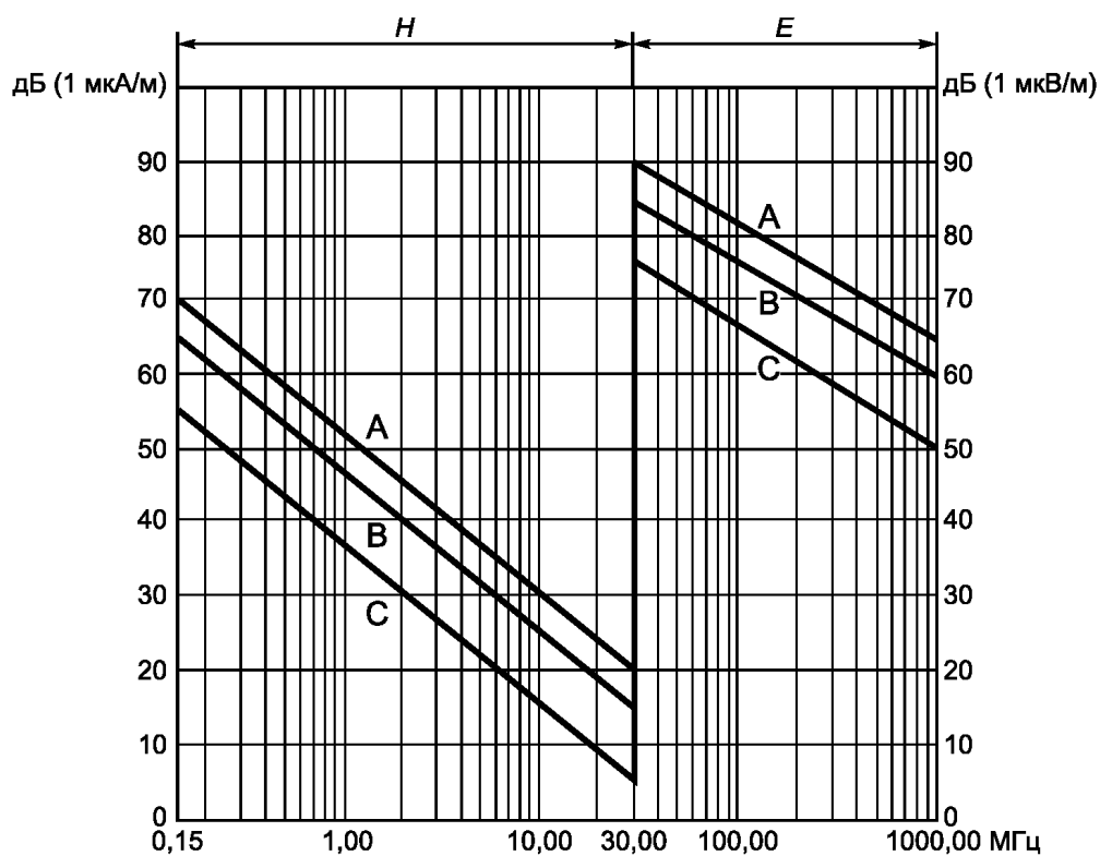
Кривая А — при питании подвижного состава от сети переменного тока напряжением 25 кВ; кривая В — при питании подвижного состава от сети постоянного тока напряжением 3 кВ; кривая С — для автономного подвижного состава
