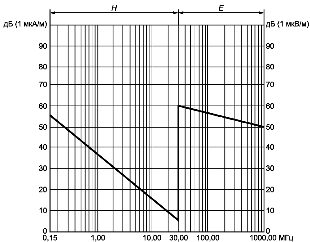
Рисунок 1 — Нормы напряженности поля электромагнитных помех (квазипиковые значения), создаваемых подвижным составом на стоянке
