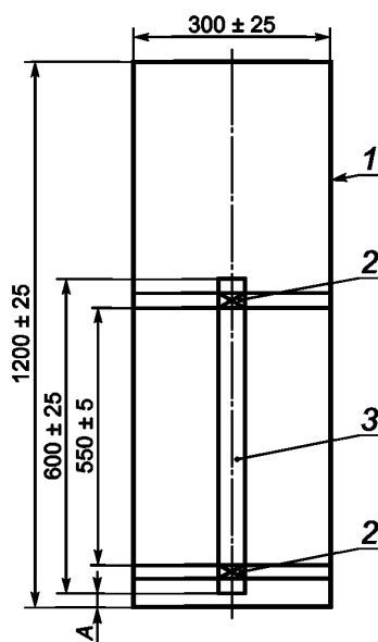
1 — металлическая камера; 2 — опорный стержень и крепление медной проволокой; 3 — образец; A — расстояние от дна камеры до нижнего конца образца (около 50 мм)
