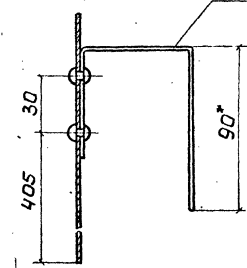
В-В M 1:2
