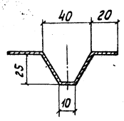
III M 1:2
