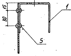
A-A M 1:2
