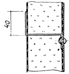
Б-Б M 1:2
