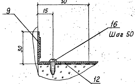
Разрез Д-Д лист 8
