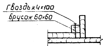
Сечение 10-10
