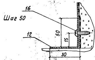
Сечение Е-Е лист 8
