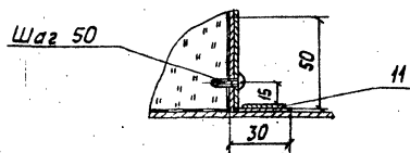
Сечение З-З лист 4
