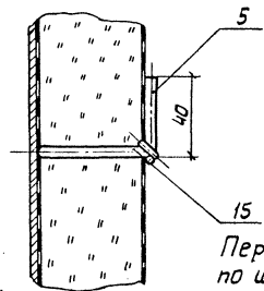
Сечение А-А лист 8
