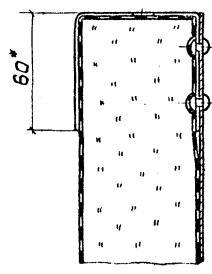
А-А M 1:2
