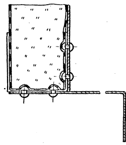
Е-Е M 1:2
