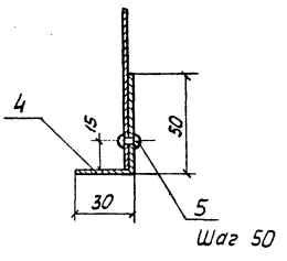
B-B M 1:2
