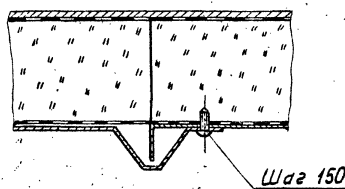
Сечение Д-Д лист 4
