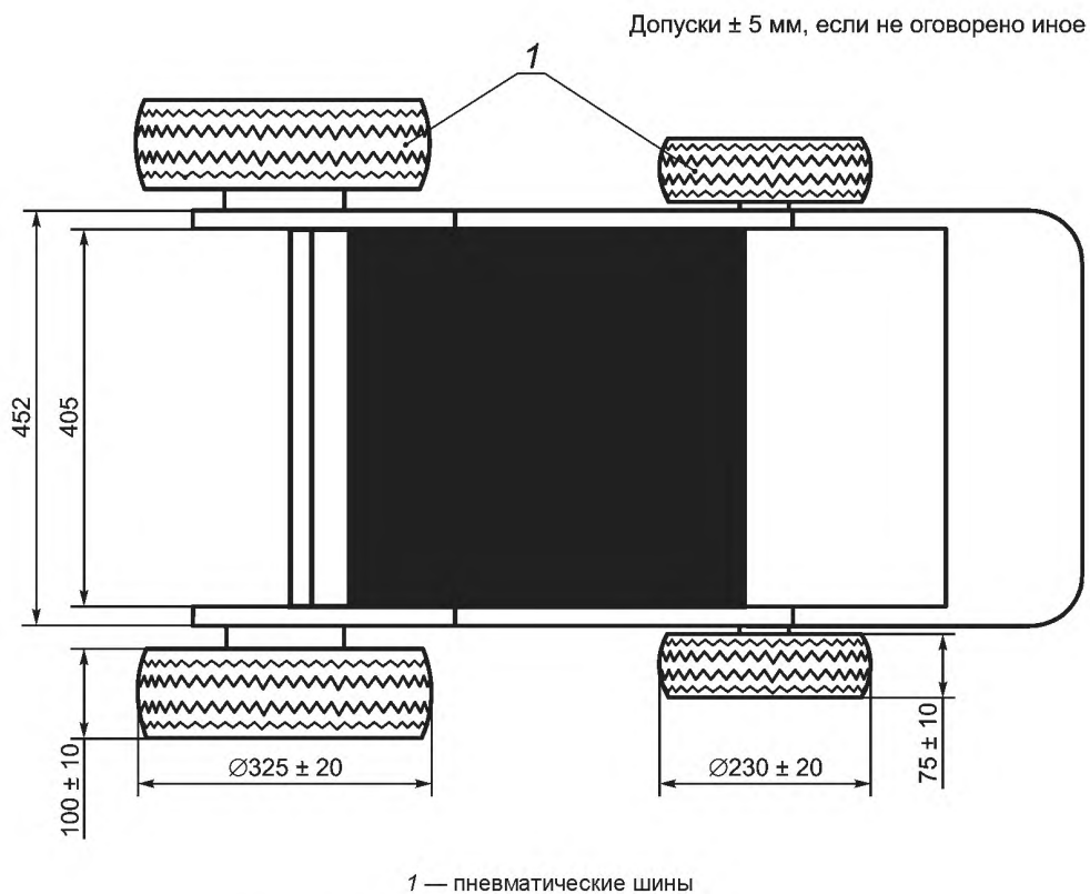
Рисунок Е.3 — Имитатор кресла-коляски, вид сверху
