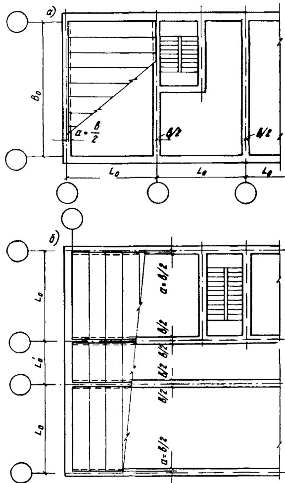
Рис. 4. Примеры привязки стен к модульным разбивочным осям в плане здания с несущими стенами
