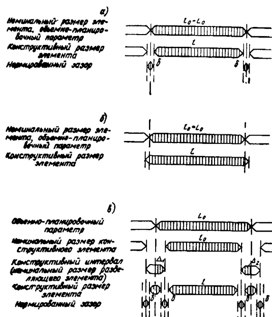
Рис. 1. Размеры элементов, применяемых в строительстве
