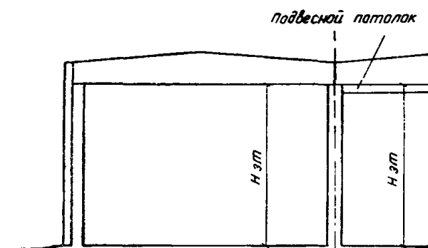
Рис. 10. Номинальный модульный размер высоты этажа в одноэтажных и многоэтажных зданиях
