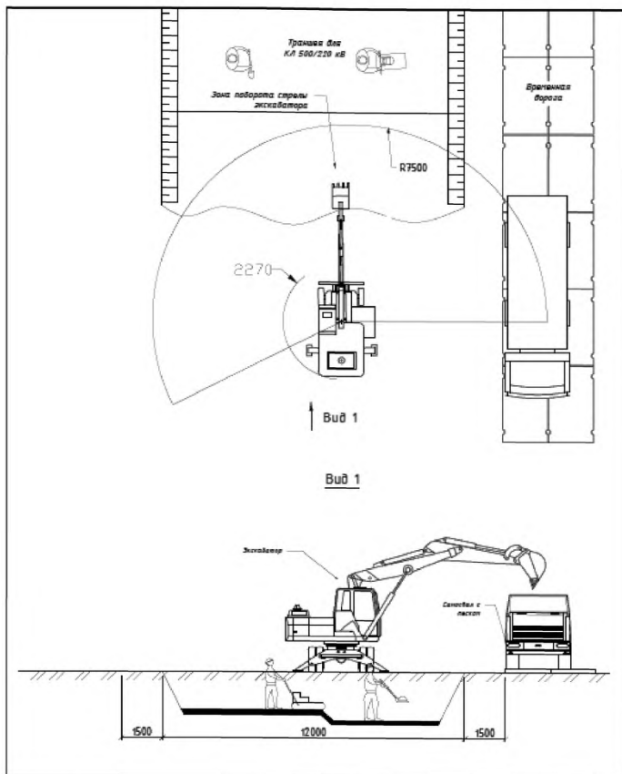
Рис. 1 Раскопка траншеи, устройство песчаной подушки с трюмбровкой
