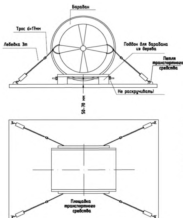
Рис. 3 Хранение кабельного барабана
