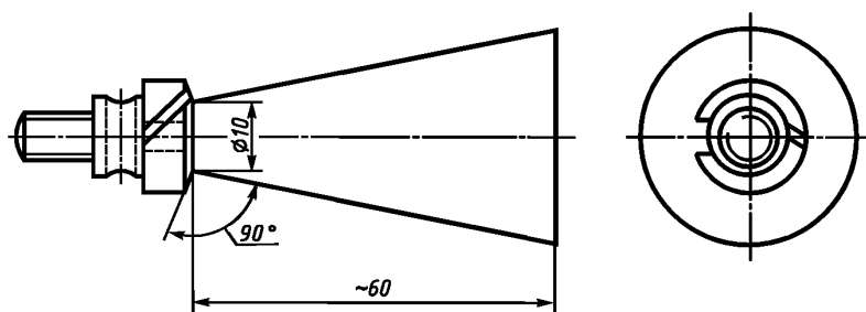
Рисунок 1 — Коническая оправка
