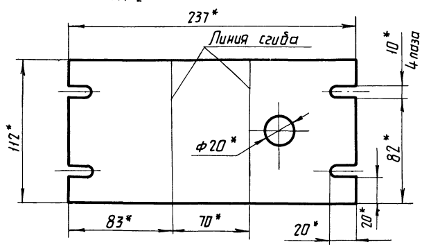
Развертка M1:2
