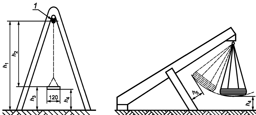
1 — ось вращения элемента подвеса (шарнир); h_1 — высота качелей; h_2 — длина элемента подвеса сиденья качелей; h_3 — высота подвески сиденья; h_4 — расстояние от сиденья до поверхности игровой площадки; h_5 — расстояние от сиденья до опорных конструкций
