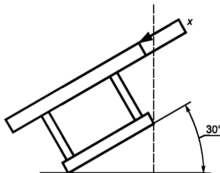
Рисунок 7 — Сиденье-колыбель
