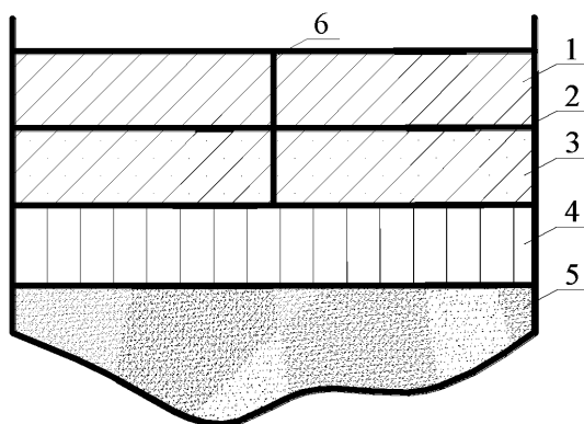
Рис.5. 5. Усиление цементобетонного покрытия методом сращивания:
