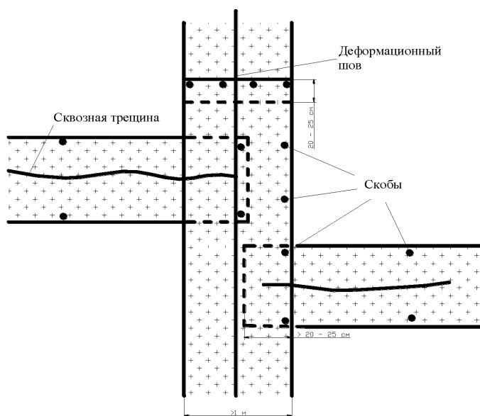
Рис. 5.3. Схема локального армирования геосинтетическими материалами
