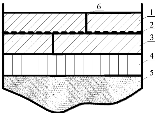
Рис.5.6. Усиление цементобетонного покрытия методом наращивания:
