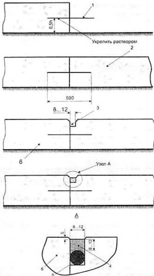
Рис.4.5. Конструктивная схема ложного шва: 1 - металлический анкер; 2- свежееуложенный бетон; 3- паз для герметика; 4 - герметик; 5 - уплотнительный шнур; 6 - смежная плита.
