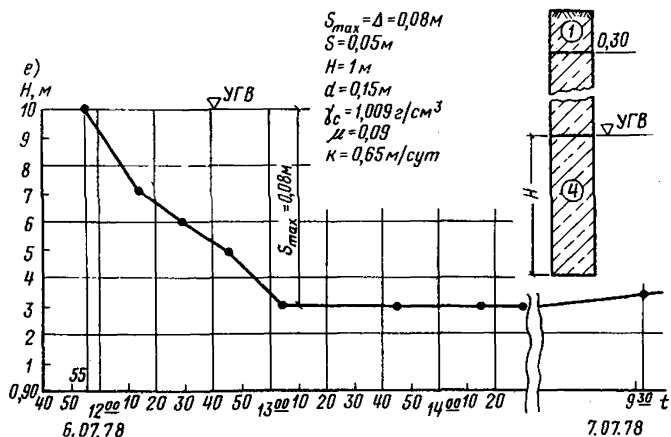
Рис. 7. Результаты проведения опытно-фильтрационных работ методом тяжелой жидкости на объектах изысканий
