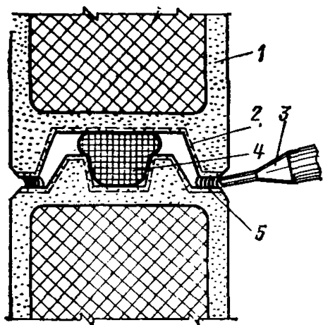
Рис. 34. Изоляция стыка между стеновыми панелями с укладкой мастичного герметика на боковые поверхности гребней панелей до их монтажа
