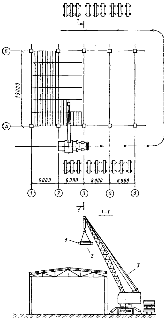
Рис. 18. Схема монтажа плит покрытия из ПАЭ комплексным методом
