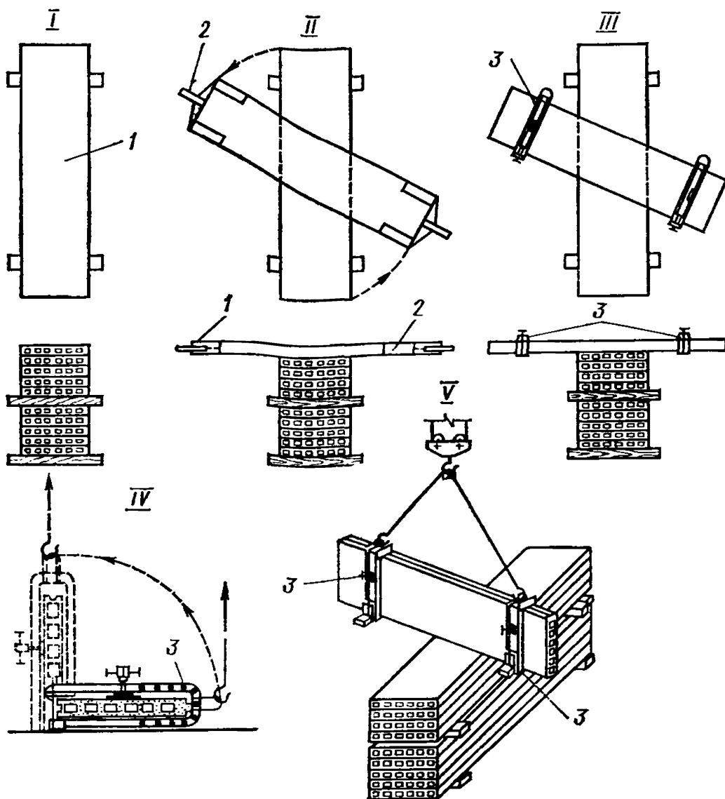
Рис. 12. Схема строповки панелей при поэлементном монтаже стен горизонтальной разрезки
