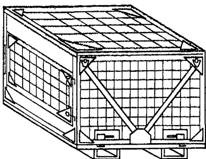
Рис. 21. Контейнер КЗ—1Г ЦНИИОМТП для рулонных материалов
