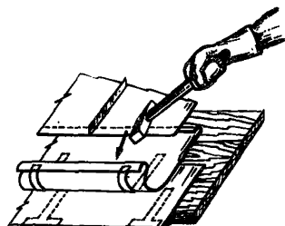
Рис. 3. Отгибание крюков и желоба
