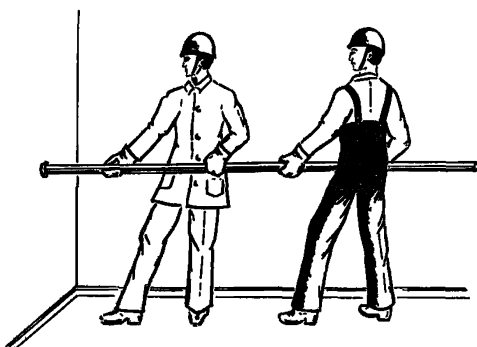
Рис. 53. Освобождение трубы из стены
