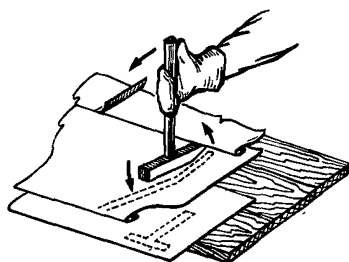
Рис. 4. Отгибание лежащего фальца у желоба
