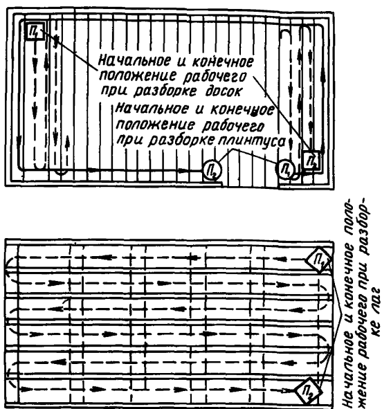
Рис. 29. Схема организации рабочего места
