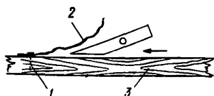
Рис. 8. Удаление кляммеры 1—гвоздь; 2—кляммера; 3—обрешетка
