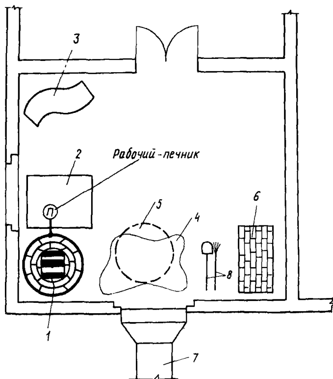
Рис. 43. Схема организации рабочего места 1—разбираемая печь; 2—переносные инвентарные подмости; 3—место складирования листов футляра; 4—строительный мусор; 5—место окучивания мусора; 6—штабель годного кирпича; 7—желоб (лоток) для спуска мусора; 8—лопата совковая или прутяная метла
