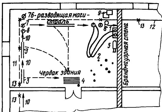
Рис. 48. Схема организации рабочего места 1—баллоны ацетиленовый и кислородный; 2—шланги ацетиленовый и кислородный; 3—демонтированные участки труб; 4—место складирования отрезков труб; 5—тележка для баллонов с газом; 6—слесарь-сантехник I разряда; 7—слесарь-сантехник II разряда; 8—ведро с водой; 9—асбестовые листы; 10—направление движения; 11—демонтированная магистраль; 12—существующая разводящая магистраль; 13—стойка
