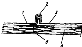
Рис. 5. Схема крепления кровельных листов кляммерами к обрешетке 1—верхний лист; 2—кляммера; 3—нижний лист; 4—обрешетка; 5—гвоздь
