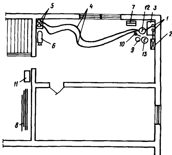
Рис. 54. Организация рабочего места 1—демонтируемые стояки; 2—радиатор; 3—асбестовый лист; 4—шланги ацетиленовый и кислородный; 5—баллоны с газом; 6—тележка для перевозки баллонов; 7—ящик для инструментов; 8—пакет складываемых демонтированных участков труб; 9—ведро с водой; 10—кисть; 11—ящик для снятых креплений стояков; 12—газорезчик IY разряда; 13—слесарь-сантехник II разряда
