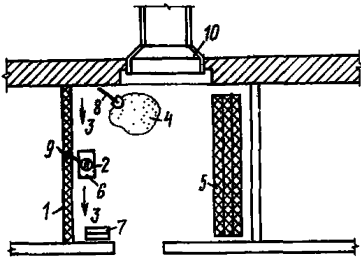
Рис. 34. Схема организации рабочего места
