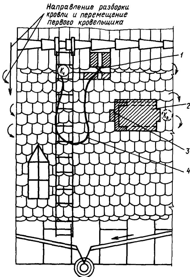
Рис. 10. Схема организации рабочего места K_1 —положение первого кровельщика на кровле; K_2 — позиция второго кровельщика на чердаке; 1—крепле- ние страховочной веревки; 2—проем для спуска чере- пицы на чердак; 3—желоб (лоток) для спуска чере- пицы; 4—страховочная веревка
