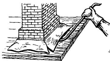
Рис. 15. Удаление покрытия из кровельного железа в примыкании кровли к дымовой трубе
