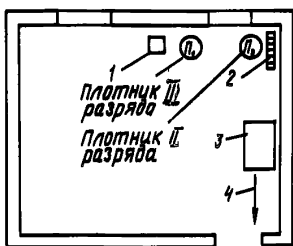
Рис. 39. Схема организации рабочего места 1—ящик для инструмента; 2—лестница-стремянка; 3—место временно-го складирования; 4—направление откоски
