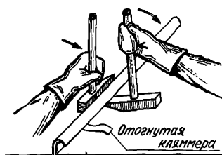
Рис. 2. Разгибание стоячего фальца
