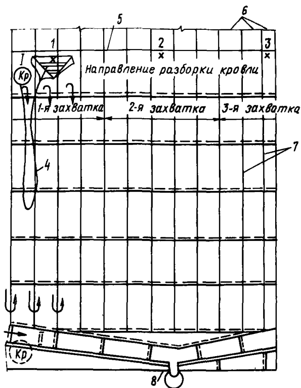
Рис. 1. Схема организации рабочего места 1, 2, 3, х—порядок переноса и место крепления страховочной веревки; Кр—1; П—положение и последовательность перемещения кровельщика; 4—страховочная веревка; 5—конек; 6—ряды кар- тин; 7—стоячие фальцы; 8—карниз
