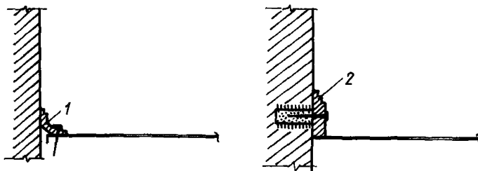
Рис. 27. Примыкание галтелей и плинтусов к стене 1—галтель; 2—плинтус
