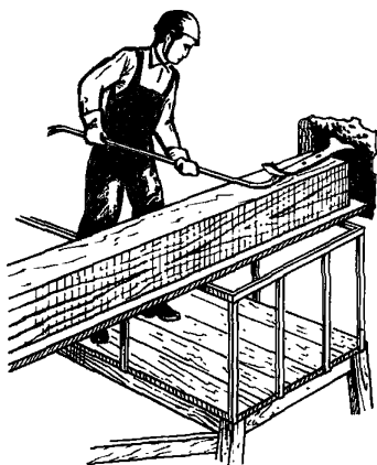
Рис. 23. Освобождение балки от анкера
