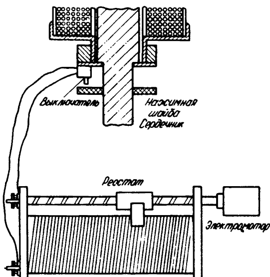
Рис. 4. Устройство для автоматической регистрации момента отрыва штампа от грунта в приборе УИЛ-2
