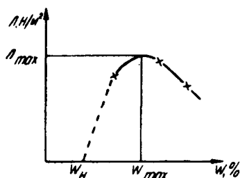
Рис. 1. Зависимость липкости грунта от его влажности
