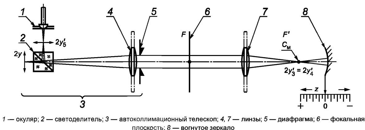
Рисунок А.1 — Установка для поверки пробной очковой линзы
