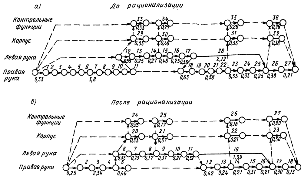
Рис. 3. Графическая модель приемов труда при укладке кирпича в ложковый ряд наружной версты
