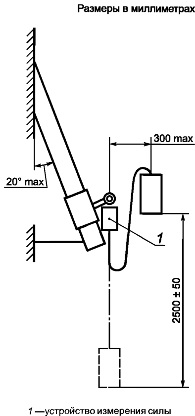
Рисунок 9 — Проверка динамической характеристики анкерных устройств, закрепляемых на наклонных крышах
