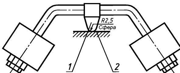
1 — стальной шарик; 2 — испытываемая поверхность Рисунок 6 — Устройство для испытания вдавливанием шарика
