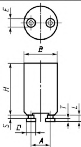
Рисунок 1 — Размеры стартеров
