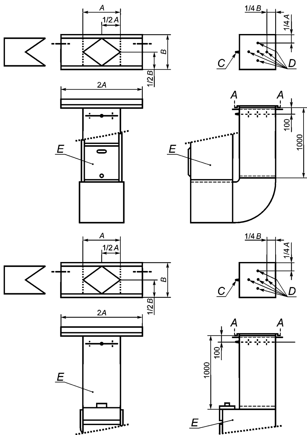
A и B — размеры выпускных отверстий; C — место измерения статического давления воздуха; D — место измерения температуры воздуха на поверхности корпуса; E — аппарат
