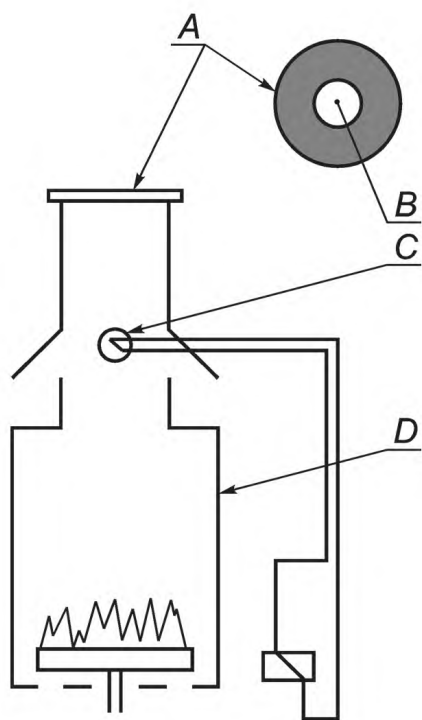
A — пластина с отверстием; B — отверстие площадью 35 % от номинальной площади сечения дымохода; C — датчик системы безопасности, контролирующей поступление продуктов сгорания в помещение; D — аппарат
