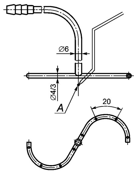
А — термопара
