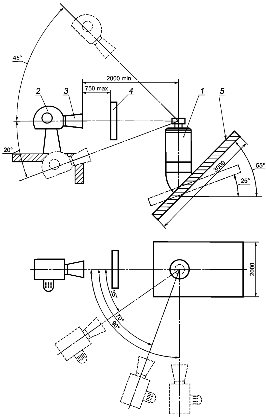
1 — подача воздуха для горения и отвод продуктов сгорания; 2 — генератор воздушного потока (должен обеспечить установленные скорости воздуха по всему фронту воздушного потока с точностью \pm 10\% ); 3 — диффузор; 4 — фронтальная перегородка воздушного потока (должна быть такой, чтобы полностью перекрыть входное и выпускное отверстия наконечника); 5 — испытательная поверхность
