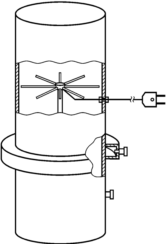
Рисунок 9 — Пробоотборник для аппаратов типа С 6
