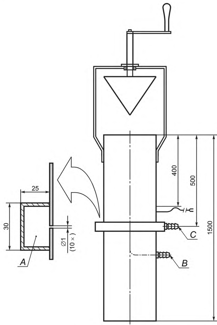
А — кольцевая камера с 10 отверстиями диаметром 1 мм для измерения статического давления; В — место отбора проб продуктов сгорания; С — место измерения статического давления
