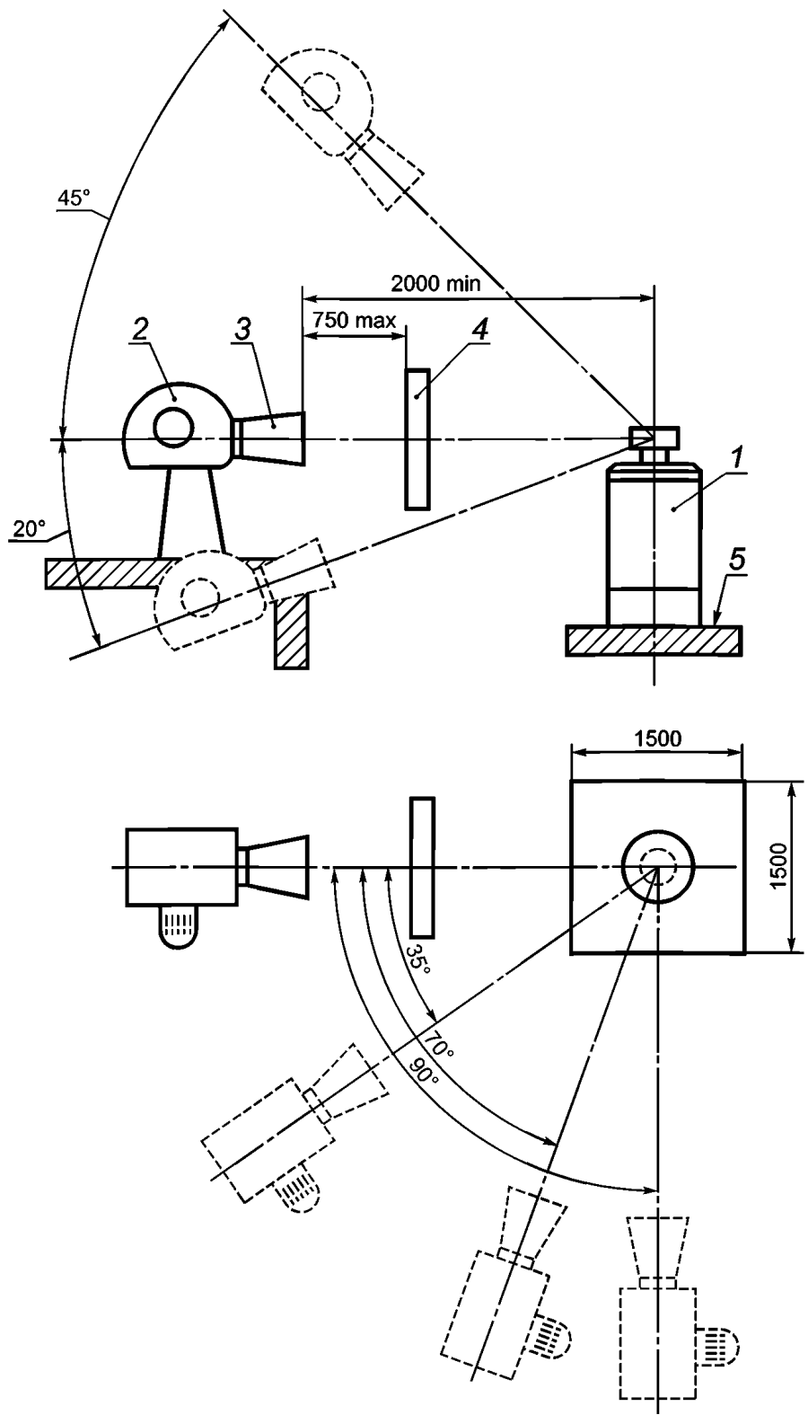
1 — подача воздуха для горения и отвод продуктов сгорания; 2 — генератор воздушного потока (должен обеспечить установленные скорости воздуха по всему фронту воздушного потока с точностью \pm 10\% ); 3 — диффузор; 4 — фронтальная перегородка воздушного потока (должна быть такой, чтобы полностью перекрыть входное и выпускное отверстия наконечника); 5 — испытательная поверхность
