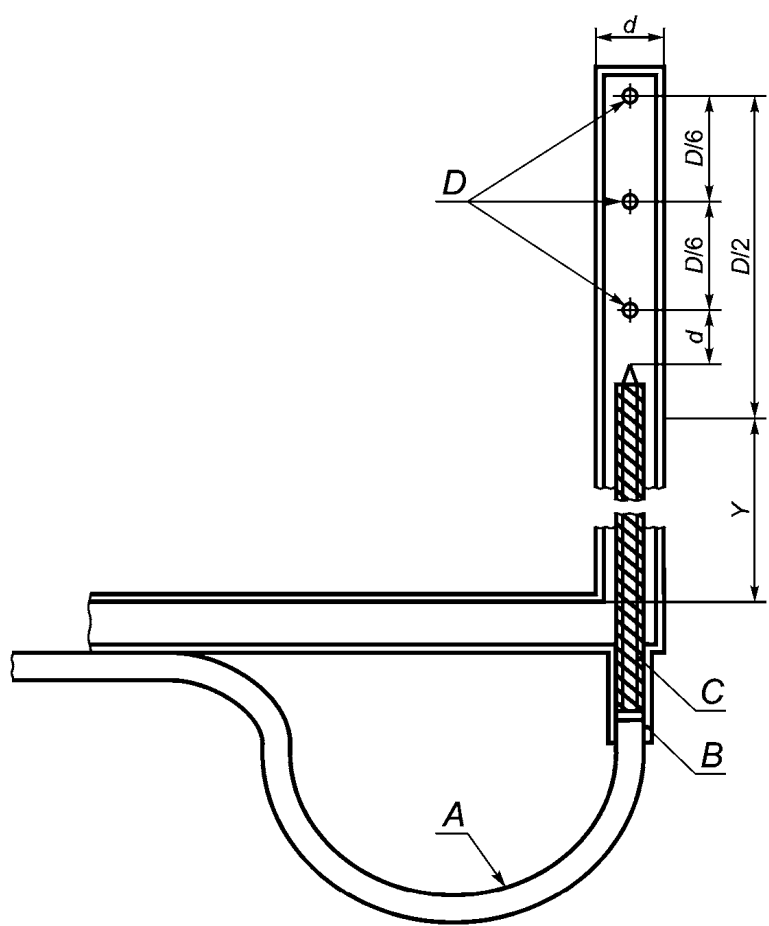
А — провод хромоалюминиевой термопары; В — изолирующий материал; С — керамическая втулка с двойным отверстием; D — три отверстия для отбора проб Ø X мм
