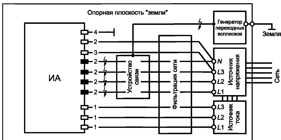
Рисунок Е.2 — Установка для проведения испытаний на устойчивость к наносекундным импульсным помехам. Цепи напряжения
