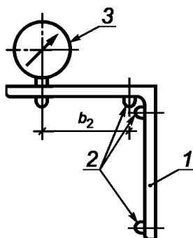
b_2 — база прибора; 1 — корпус (угольник); 2 — опора; 3 — индикатор
