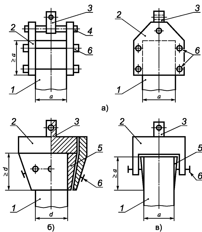
Рисунок К.2 — Схема приклеиваемых и анкерных захватов
