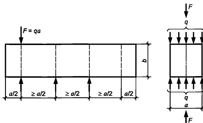
г) Образцы-призмы из тяжелого бетона
