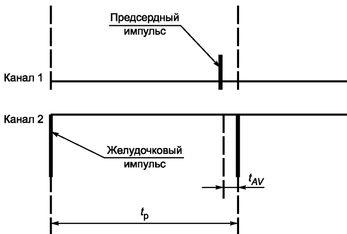
Рисунок 11 — Изображение на осциллографе при измерении A-V интервала
