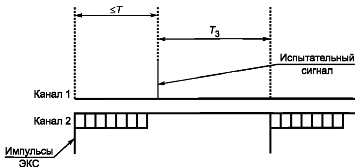
Рисунок 5 — Измерение длительности задержки ( T_3 ) у R-запрещаемого ЭКС
