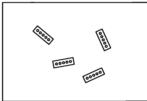
Рисунок Н.1 — Типичные положения ударной машины для напольных покрытий категорий II или III и тяжелого стандартного пола
