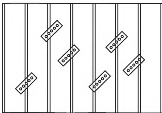
Рисунок Н.2 — Типичные положения ударной машины для напольных покрытий и легкого стандартного пола
