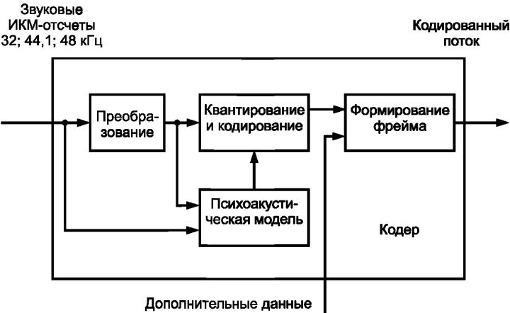
Рисунок 1 — Общая структура кодера
