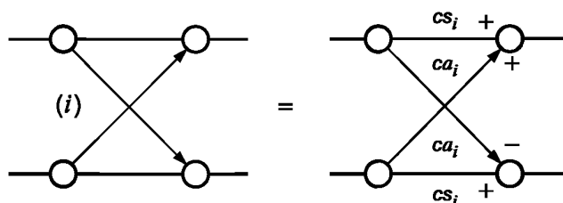
Рисунок В.8 — «Бабочка» в кодере
