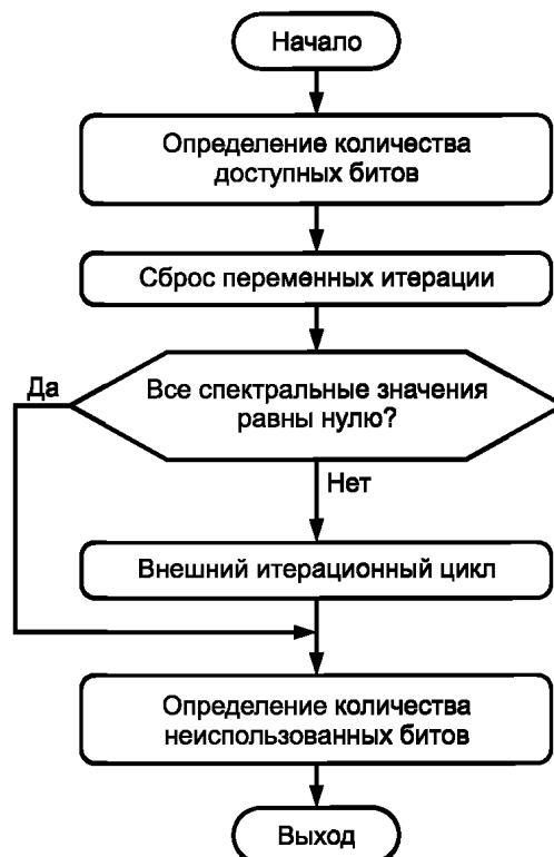
Рисунок В.9а –Цикл итерации. Уровень III.
