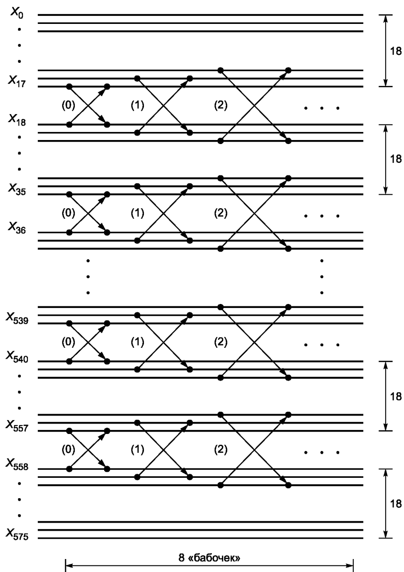
Рисунок А.5 — Диаграмма устранения элайзинга в декодере. Уровень III
