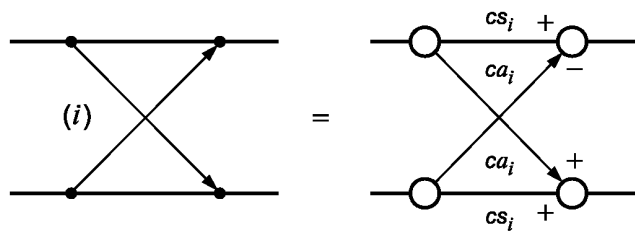
Рисунок А.6 — «Бабочка» устранения элайзинга в декодере. Уровень III
