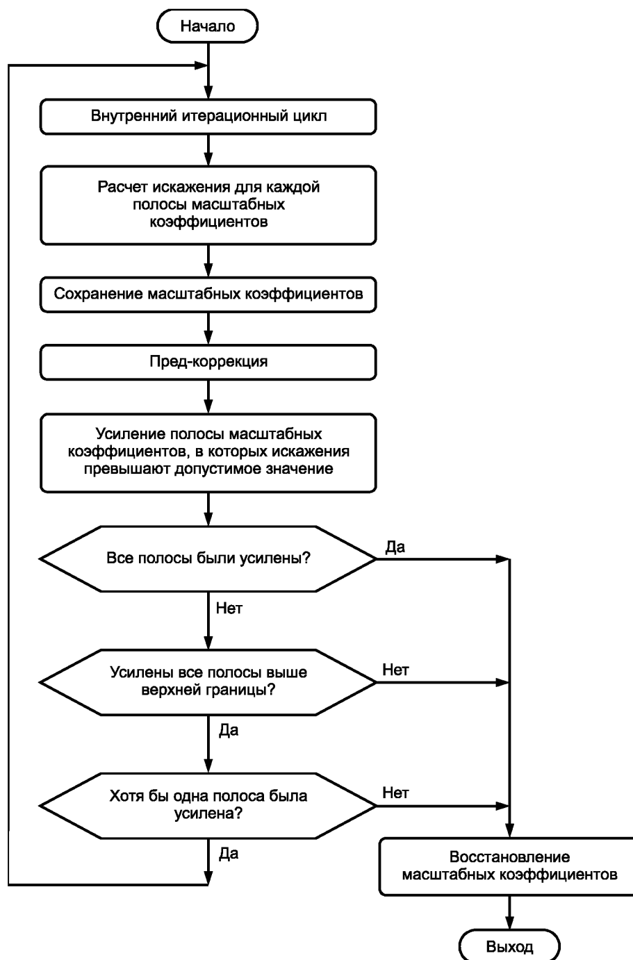
Рисунок В.9б – Внешний цикл итерации. Уровень III
