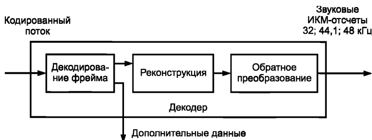
Рисунок 2 — Общая структура декодера
