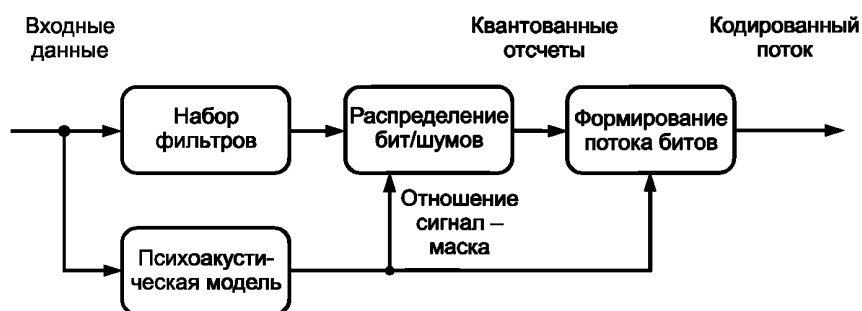
Рисунок В.1 — Блок-схема кодера
