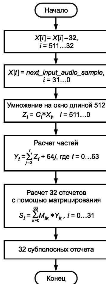
Рисунок В.4 — Блок-схема алгоритма субполосной фильтрации
