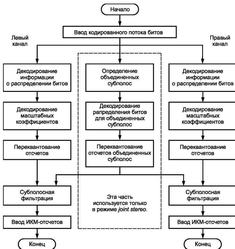
Рисунок Ж.2 — Общая блок-схема декодера стерео
