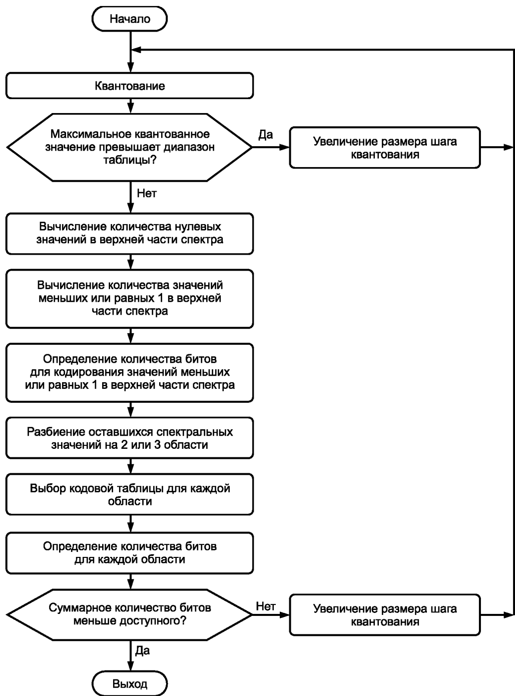
Рисунок В.9в –Внутренний цикл итерации. Уровень III
