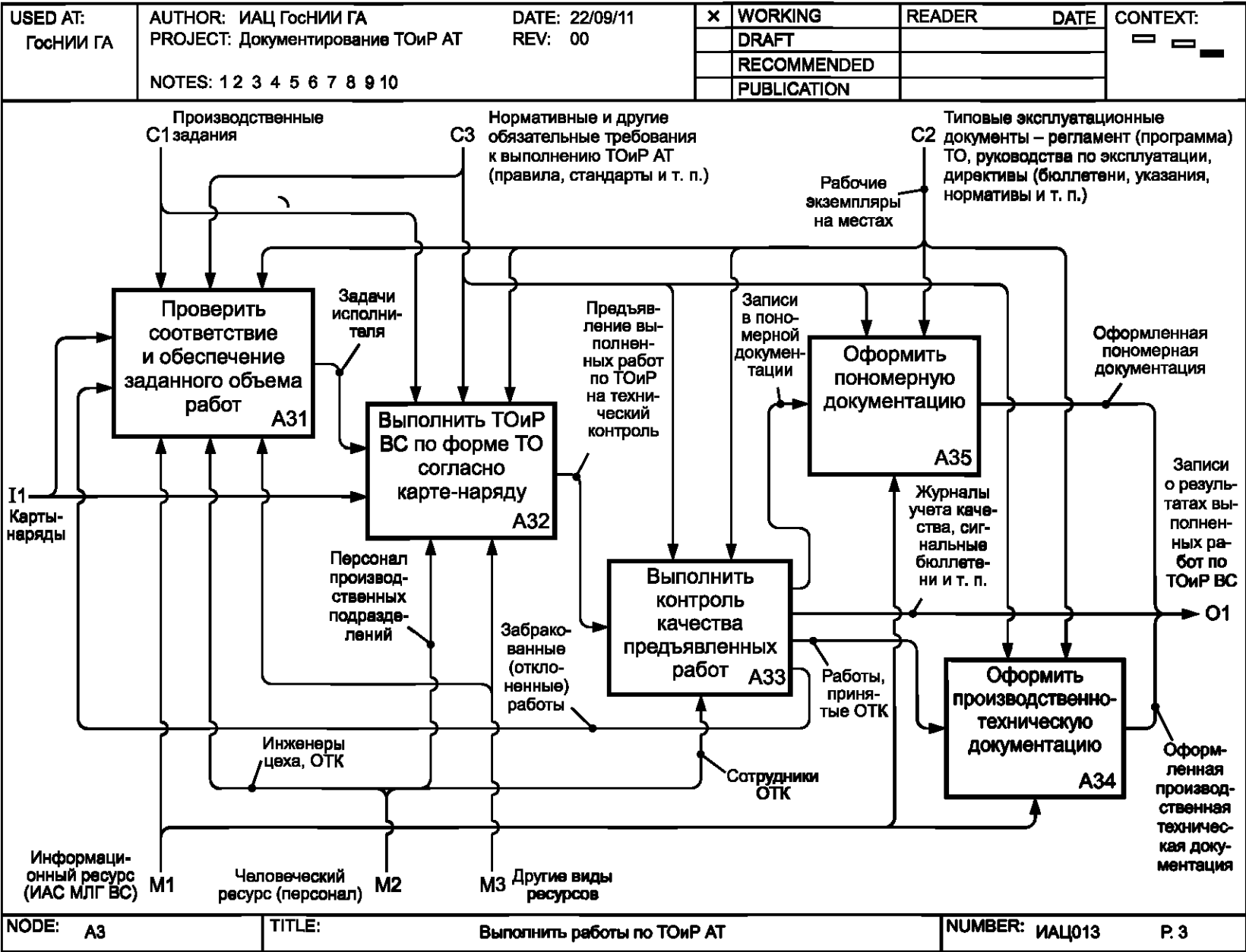
Рисунок А.2 — Алгоритм документирования ТОиР АТ
