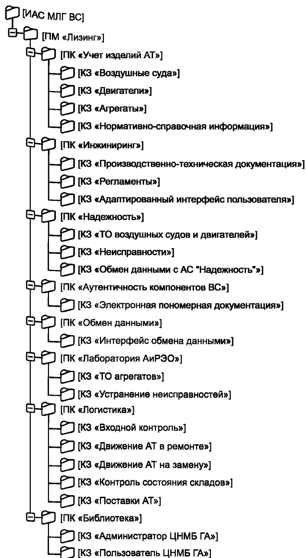
Рисунок 1 — Схема типовой структуры ПМ «Лизинг»
