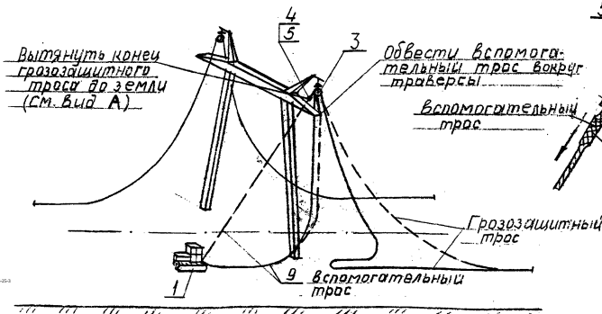
Рис. 3-1. Подъем грозазащитного троса на промежуточную опору 1-Трактор Т-130м; 2-ролик-кош на скобе СК-12; 3-ролик раскаточный МР-7; 4-монтажный захват МК-3; 5-скоба СК-7; 6-скоба СКТ-7; 7-звено промежуточное ПТМ-7; 8-трос СКХ-1,4 200; 9-трос \phi 9,6 мм \rho=100 М.
