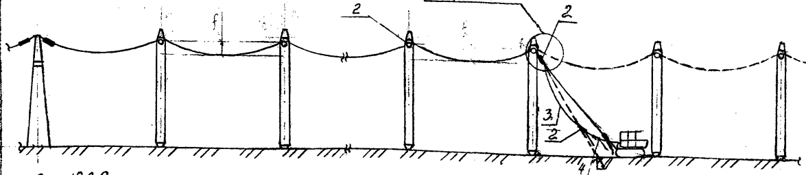
Рис 18-2 Схема натяжения и визирования грозозащитного троса в пролете ограниченного анкерно-угловой и промежуточной опорами
