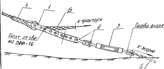
Рис. 18-4 Крепление талевых тросов при регулировке стрелы провеса грозозащитного троса
