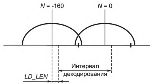
Рисунок 1 — Интервал декодирования
