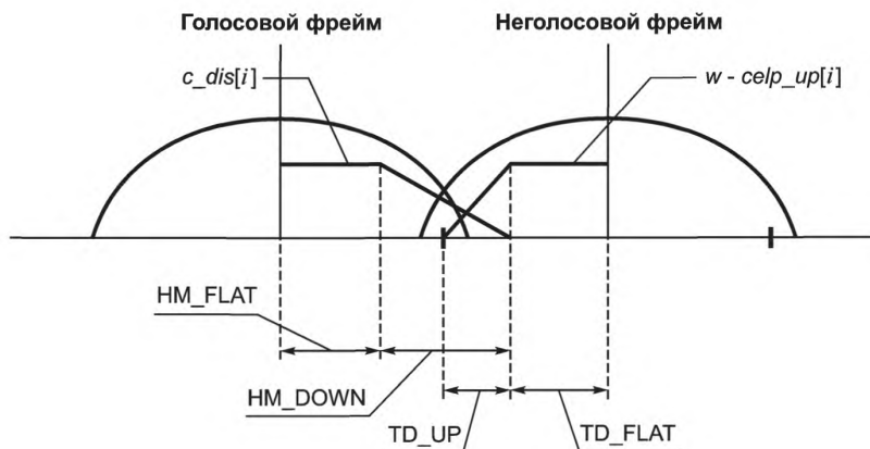
Рисунок 4 — Окно синтеза для случая речевой/неречевой
