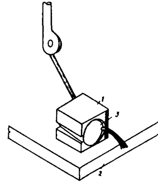
Рис.4. Клиновой зажим для закрепления начала или конца нити
