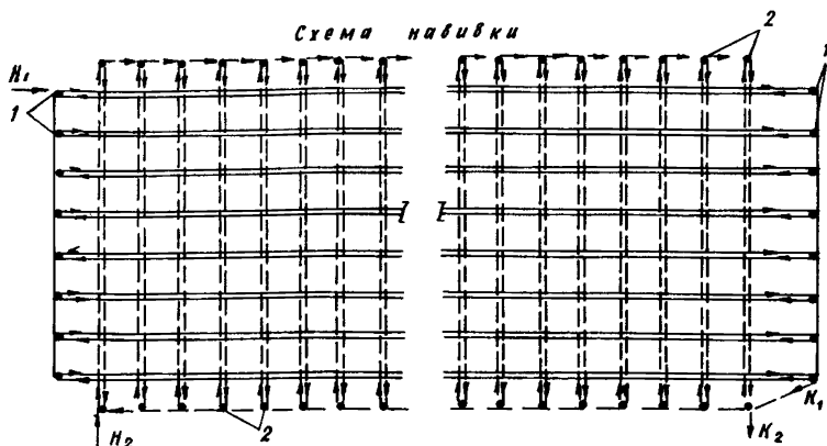
Рис.7. Схема навивки арматурной нити в двух направлениях: — в продольном; - - - в поперечном. Стрелками указано направление навивки
