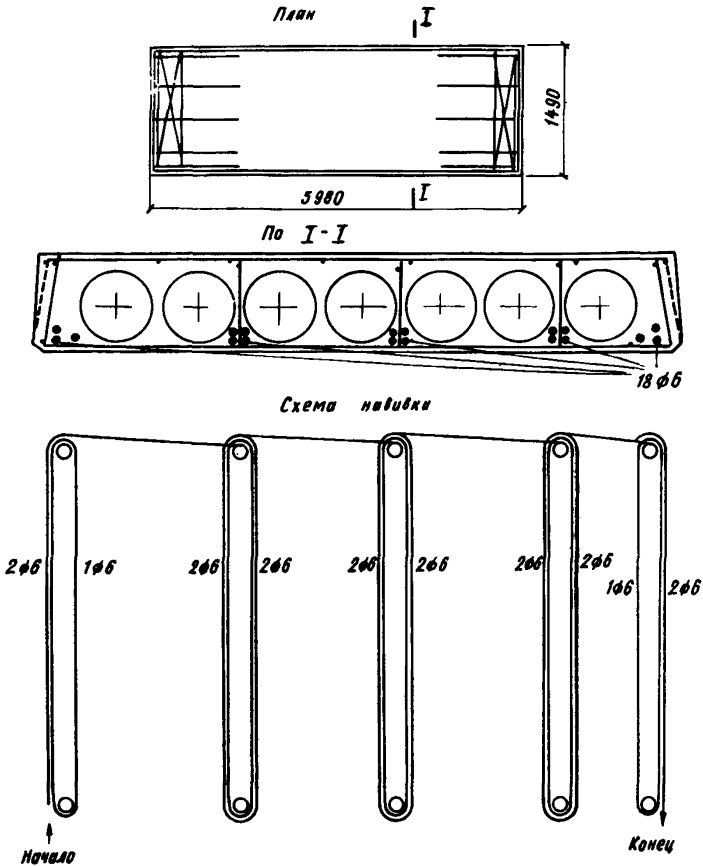
Рис.6. Схема навивки арматурного каркаса при изготовлении многопустотной панели перекрытия ПК-60.15-8К-7Т
