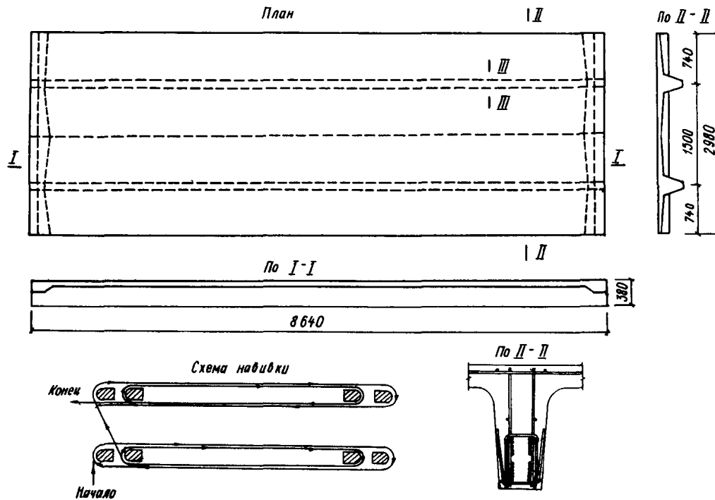
Рис. 8. Схема навивки арматурного каркаса плиты 2Т(87-30-16)
