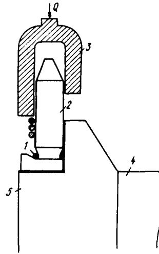
Рис.3. Закрепление конца навивки 1 - арматура; 2 - упор; 3 - пуансон; 4 - поддон; 5 - тело упора
