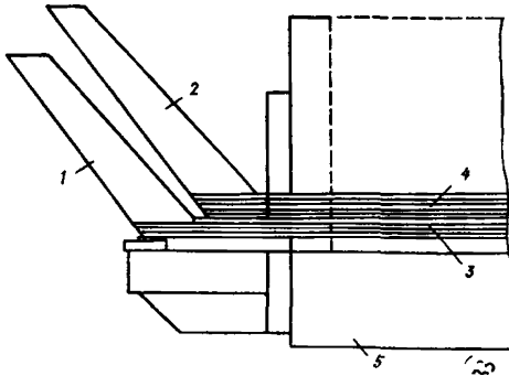
Рис.10. Стационарный упор наружного типа, так называемый "двурогий" упор.
