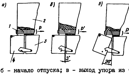
Рис.12. Упор жестко закрепленный на шарнирной части поддона. Для отпуска натяжения арматуры открывается затвор шарнирной приставки 4 (1 - арматура, 2 - изделие, 3 - поддон).
