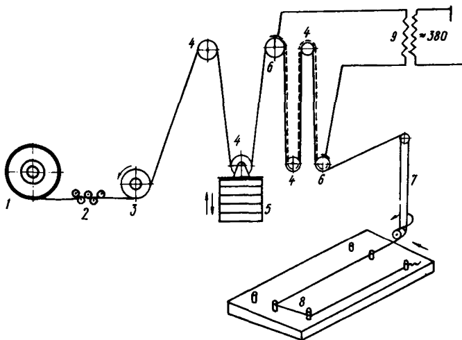
рис.1. Схема арматурно намоточного агрегата
