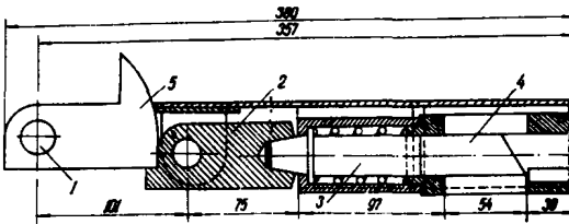
Рис.13. Упор с пружинным спусковым устройством. При отпуске натяжения клин 4 выводится из пружинного фиксатора 3, что позволяет вывести поворотный стопор 2 из зацепления с головкой фиксатора. За счет натяжения арматуры упор 5 поворачивается вокруг шарнира I
