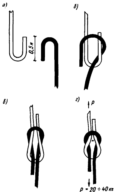
Рис.5. Сравнение каната морским узлом а - позиция 1; б - позиция 2; в - позиция 3; г - позиция 4
