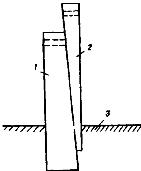
Рис.11. Упор цилиндрического типа состоит из собственно упора 1 и клина 2, вставляемых в отверстие, предусмотренное в поддоне 3, размер которого соответствует диаметру цилиндра, образованного упором и клином. Навивка арматуры производится на клин. Главная передача натяжения обеспечивается за счет удаления сначала клина, а затем упора.
