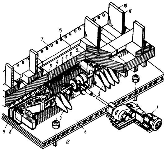
Рис.14. Наружные упоры со спускным клиновидным устройством. Применяются только при стендовой технологии для продольного армирования. Рассчитаны на восприятие усилия до 5000 кН и момента 500 кНм. Конструкция упора состоит из неподвижной плиты 6, закрепленной на фундаменте анкерными болтами 12, верхней подвижной плиты 7, на которой установлены упоры (стационарные цилиндрические или передвижные 10 с высокопрочной накладкой 11). При отпуске натяжения арматуры верхняя плита с элементами жесткости 9 (с помощью моторного или ручного привода 1, распределительного устройства 2, валов пе-
