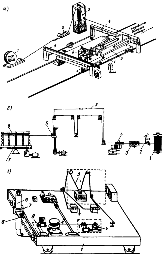
Рис. 9. Схемы устройства арматурно-намоточных агрегатов а, б - агрегаты стационарного типа (а - с координатным перемещением рабочего органа - робот, б - с вращающейся платформой); в - то же, самоходного типа
