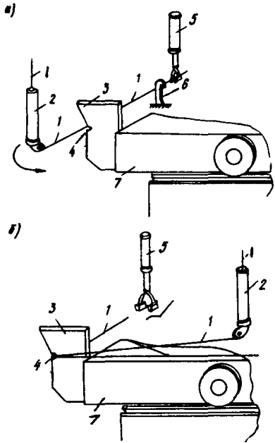
Рис.2. Закрепление начала нити при изготовлении арматурного каркаса а - начало операции; б - конец операции; 1 - арматура; 2 - пиноль; 3 - упор; 4 - кольцевая выемка; 5 - носитель арматуры; 6 - электрод; 7 - поддон
