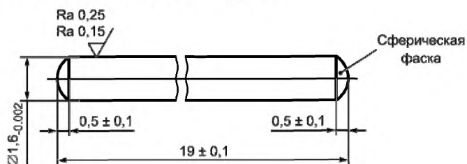
Рисунок 2 — Испытательный мандрен
